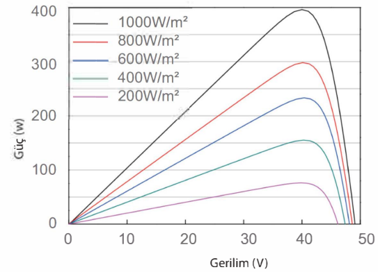
SPE 395 Güç-Gerilim Grafiği
